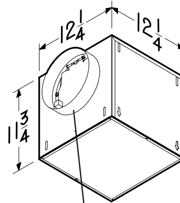
RACCORD DE CONDUIT DE 8 PO
