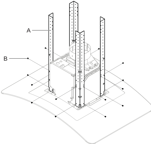
A. 4 soportes verticales superiores B. 16 tornillos de 4.2 x 8
