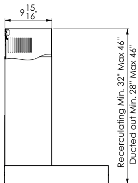
Partie latérale de la hotte
