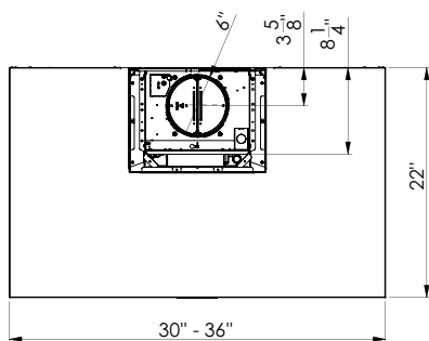
Partie supérieure de la hotte
