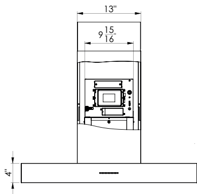
Partie avant de la hotte
