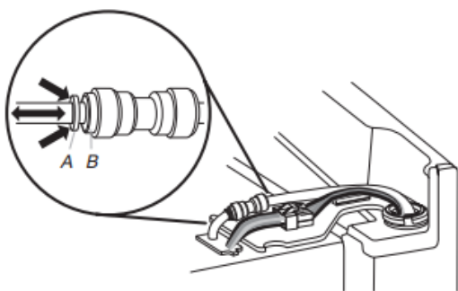
A. Bague externe
