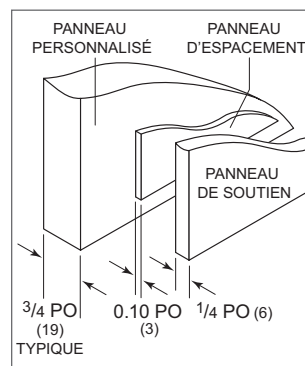
Assemblage du panneau (vue arrière)
