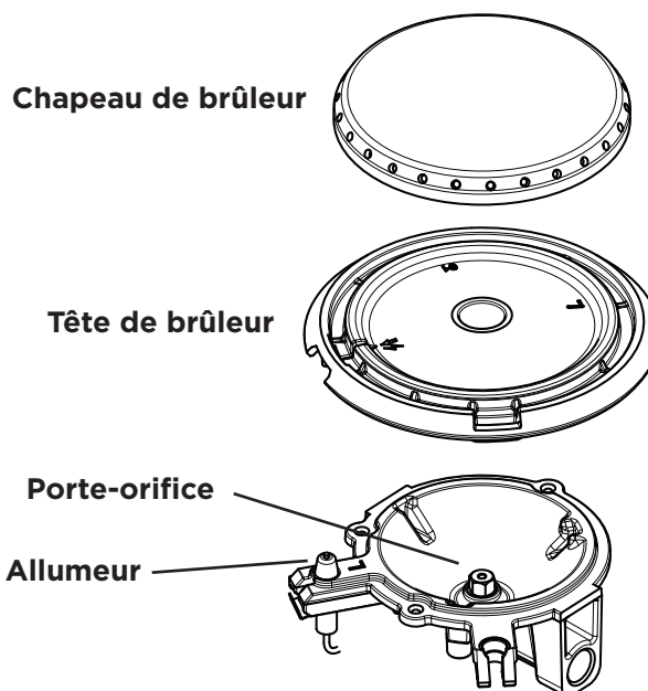
Figure 13: Composants de brûleurs scellés
