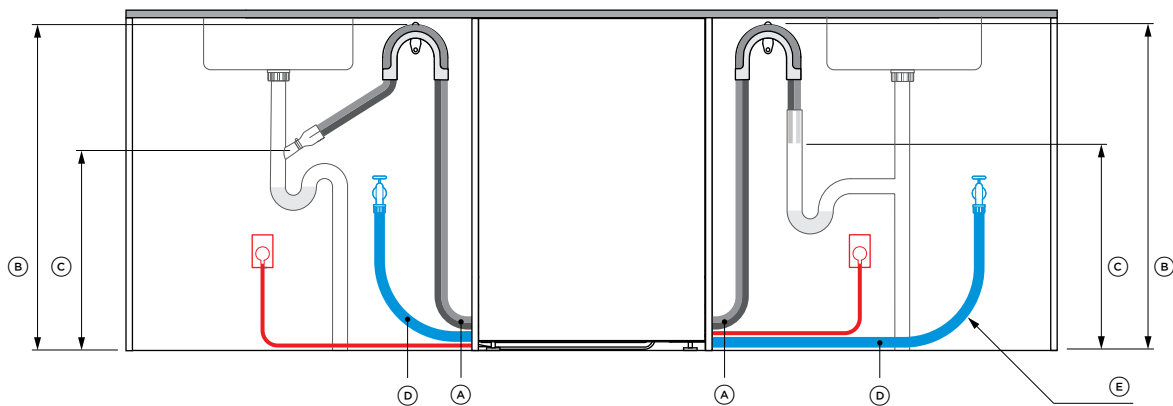
VISTA DE FRENTE INSTALACIÓN DE ESPIGA
