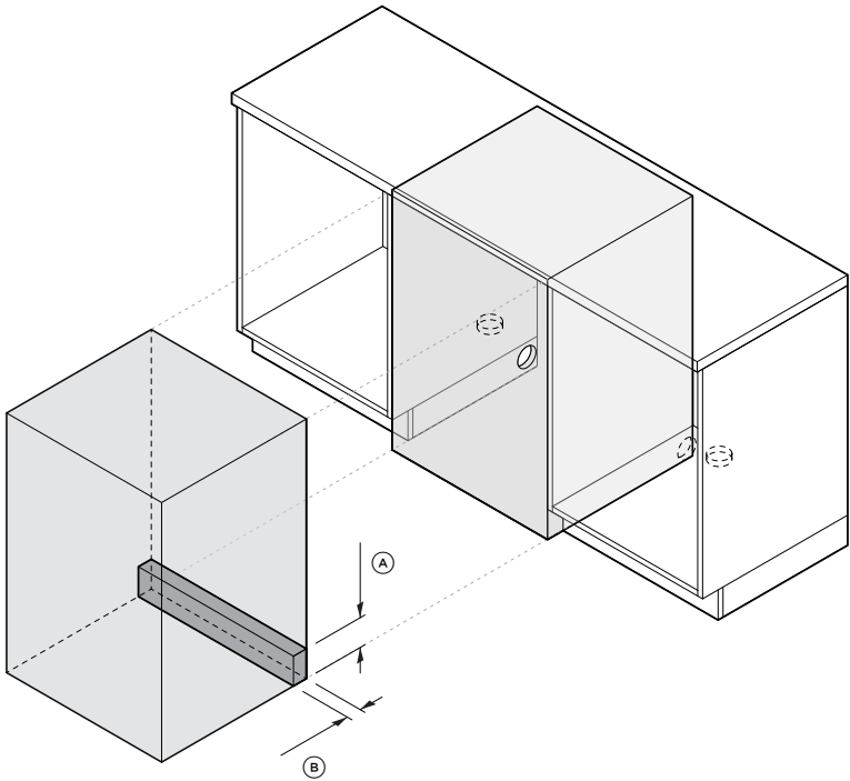
VISTA ISOMÉTRICA AMPLIADA CAVIDAD Y GABINETE
