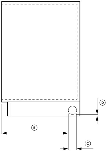
VISTA DE PERFIL GABINETES
