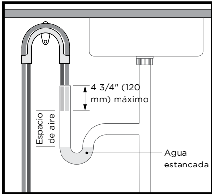
VISTA DE DETALLE INSTALACIÓN DE TUBO VERTICAL
