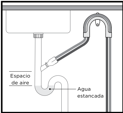
VISTA DETALLE INSTALACIÓN DE ESPIGA
