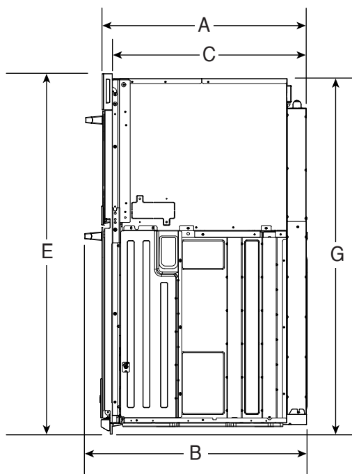
VUE LATÉRALE
