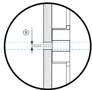
DÉTAIL 2 VUE LATÉRALE
