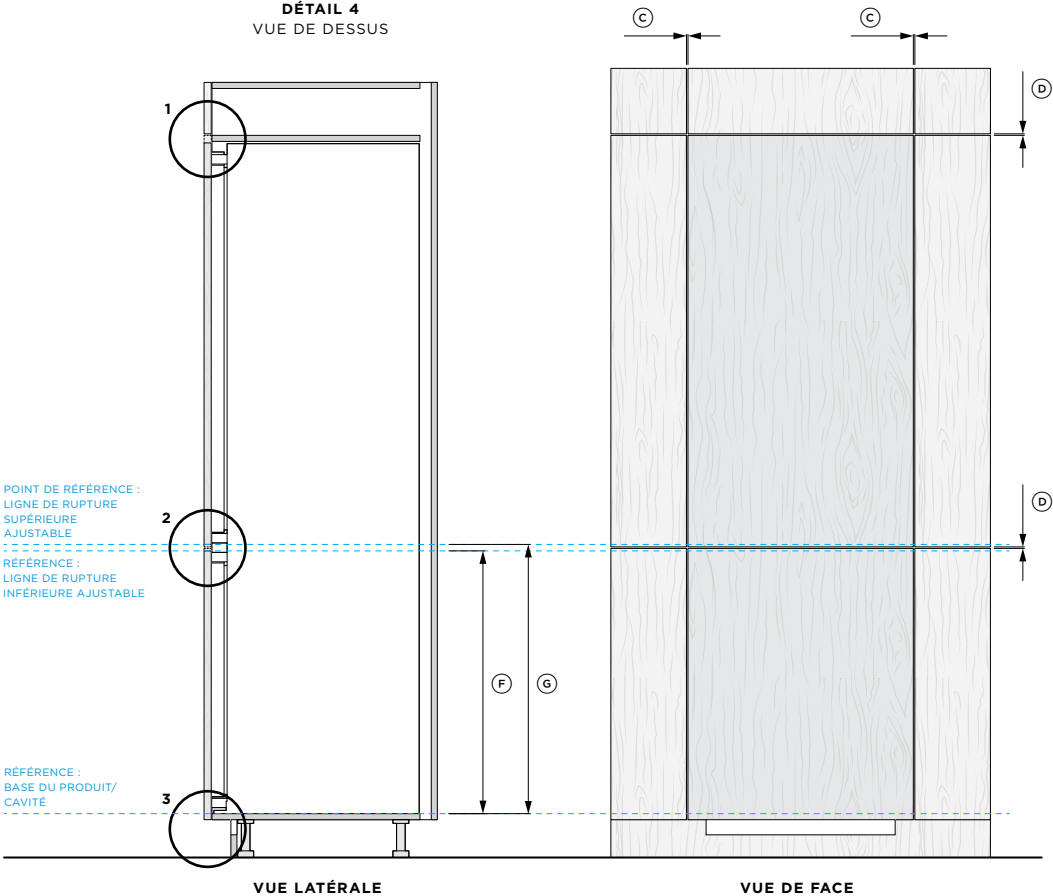
VUE LATÉRALE
