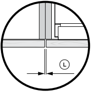
VUE EN PLAN DÉTAILLÉE PRODUIT AVEC ARMOIRES
