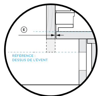
DÉTAIL 3 VUE LATÉRALE
