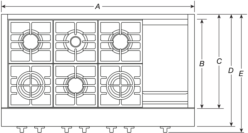
VISTA SUPERIOR
