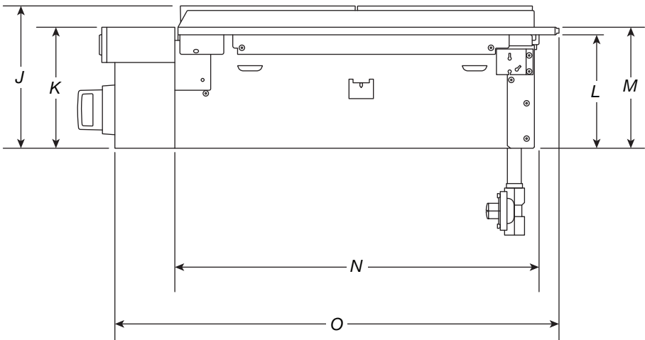
VUE LATÉRALE
