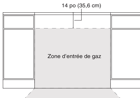
VUE AVANT
