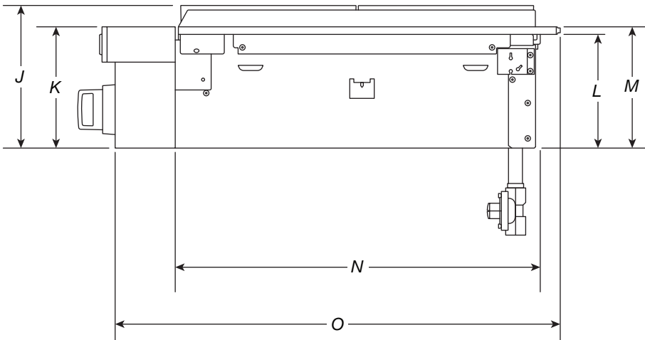
VISTA LATERAL
