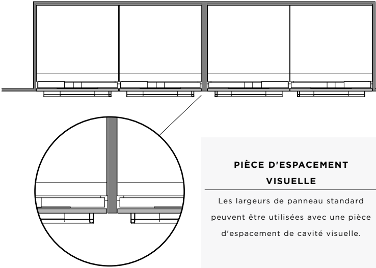
DOUBLE CAVITÉ AVEC PIÈCE D'ESPACEMENT VISUELLE
