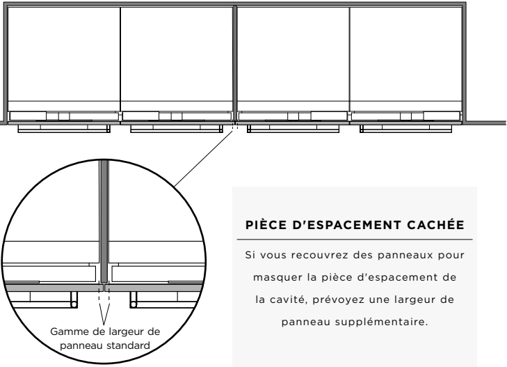
DOUBLE CAVITÉ AVEC PIÈCE D'ESPACEMENT CACHÉE
