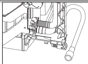
Ubicación de la manguera de desagüe
