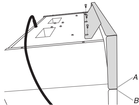
A. Bord inférieur du panneau en acier inoxydable B. Bord supérieur de la partie avant du four à micro-ondes
