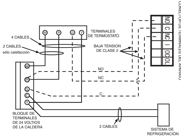
CABLEADO DE INTERBLOQUEO ALTERNATIVO DE LA CALDERA
