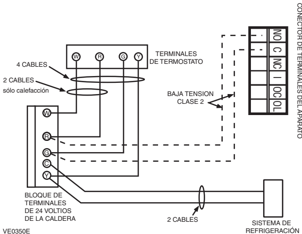
CABLEADO DE INTERBLOQUEO ESTÁNDAR DE LA CALDERA
