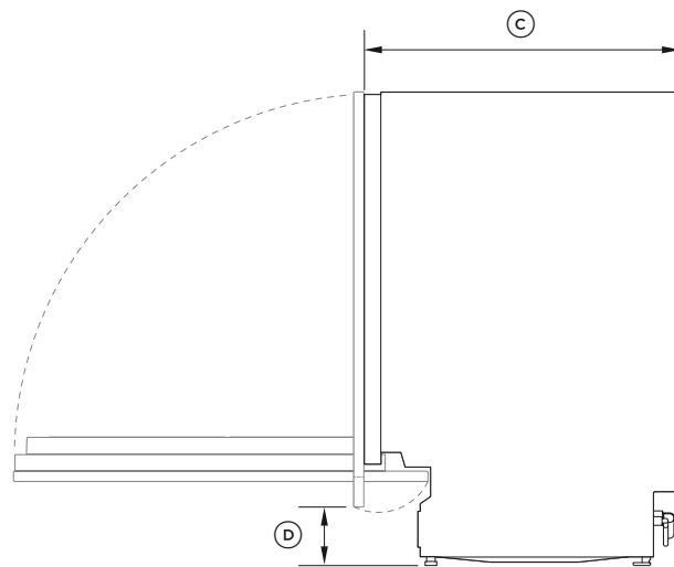
PROFIL
