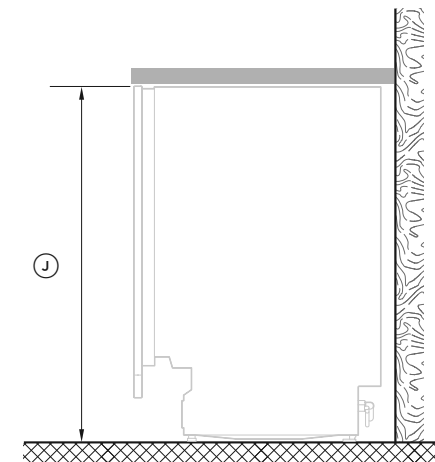
PROFIL
