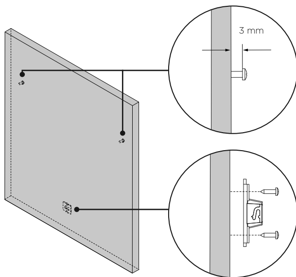
Détails de la vis supérieure (entre le panneau et la tête de vis)
