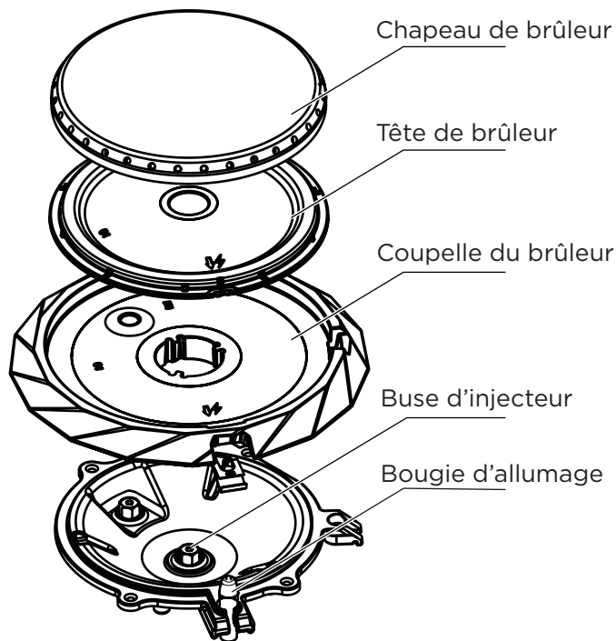
Figure 1: Ensemble Double Brûleur
