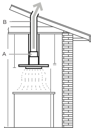
Instalaciones comunes con motor interno
