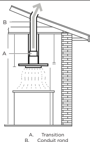
Installations typiques avec système du moteur du ventilateur interne
