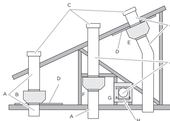
Instalaciones comunes con motor externo
