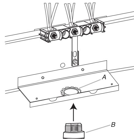
A. Tuerca de retención removible B. Conducto
