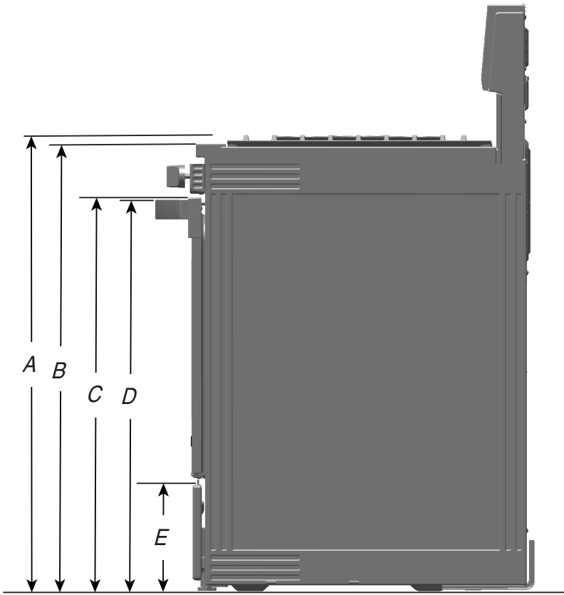
VISTA LATERAL
