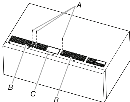
A. Tornillo B. Cubiertas de ventilaciones de recirculación C. Cubierta de iluminación de recirculación
