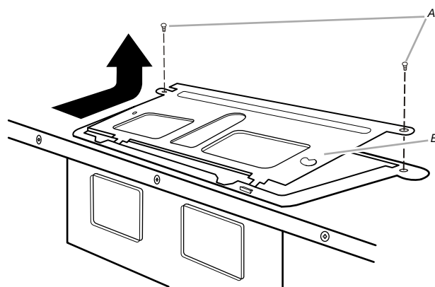
A. Tornillos B. Placa de la compuerta de tiro
