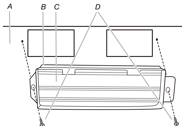
A. Parte posterior del horno de microondas B. Ensamblaje de la compuerta de tiro C. Hoja de la compuerta de tiro D. Tornillo para metal laminado de 5/32" x 5/16" (4 mm x 8 mm)
