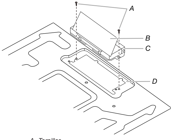
A. Tornillos B. Hoja de la compuerta C. Ensamblaje de la compuerta de tiro D. Parte superior del horno de microondas
