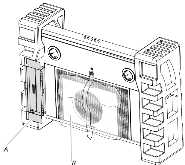
A. Transición rectangular 3 1/4" x 10" (8.3 x 25.4 cm) B. Placa de montaje redonda para ducto de escape de 7" (17.8 cm)
