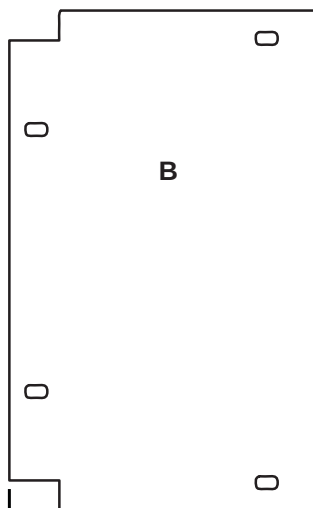
Défecteur de 11 ¾ po pour plénum de 13 po de profond
