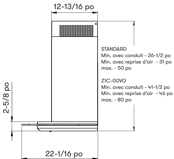
Côté de la hotte
