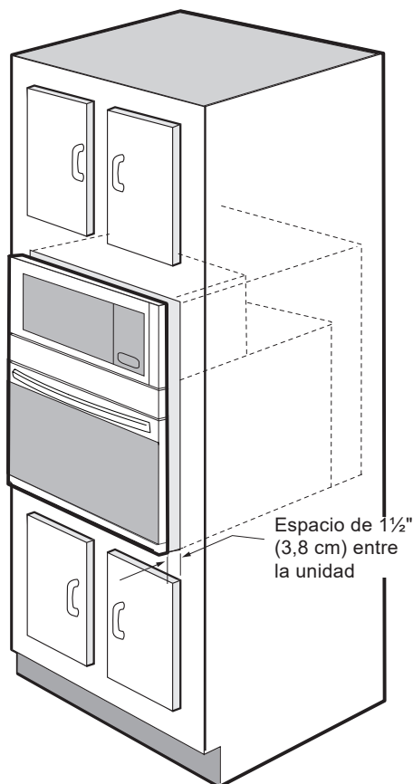
Figura 6: Instalación en el Mueble
