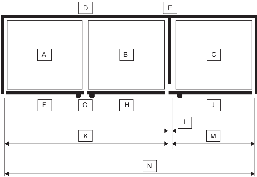
Diagrama A – Espacio Libre Más Pequeño (La Apertura de Puerta Está Restringida) Se Aplica a Paneles a Medida Únicamente.
