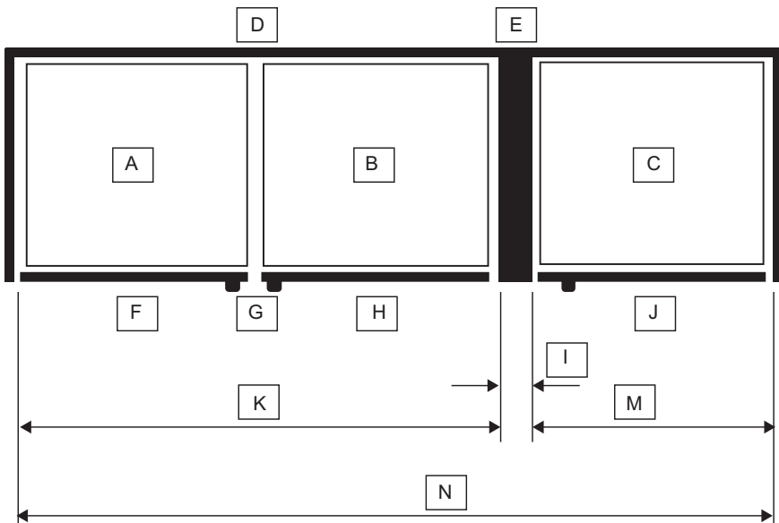
Diagrama B – Todas las Puertas se Pueden Abrir Simultáneamente Se Aplica a Paneles a Medida y de Acero Inoxidable
