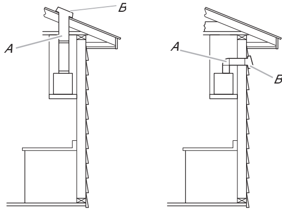
A. Conduit de dia. 6" (15,2 cm) pour décharge à travers le toit B. Bouche de décharge sur toit A. Conduit de dia. 6" (15,2 cm) pour décharge à travers le mur B. Bouche de décharge murale
