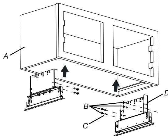
Orientation du support pour l'armoire de 30" (76,2 cm)
