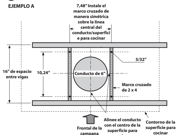
Vista superior- las vigas del techo paralelas a la parte frontal de la campana
