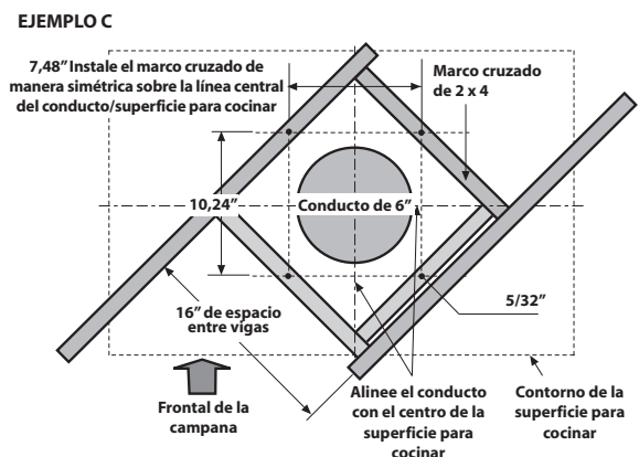
Vista superior - las vigas de la pared en ángulo con la parte frontal de la campana
