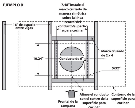
Vista superior- las vigas del techo van perpendiculares a la parte frontal de la campana
