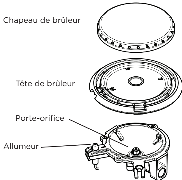
Figure 1: Brûleur unique
