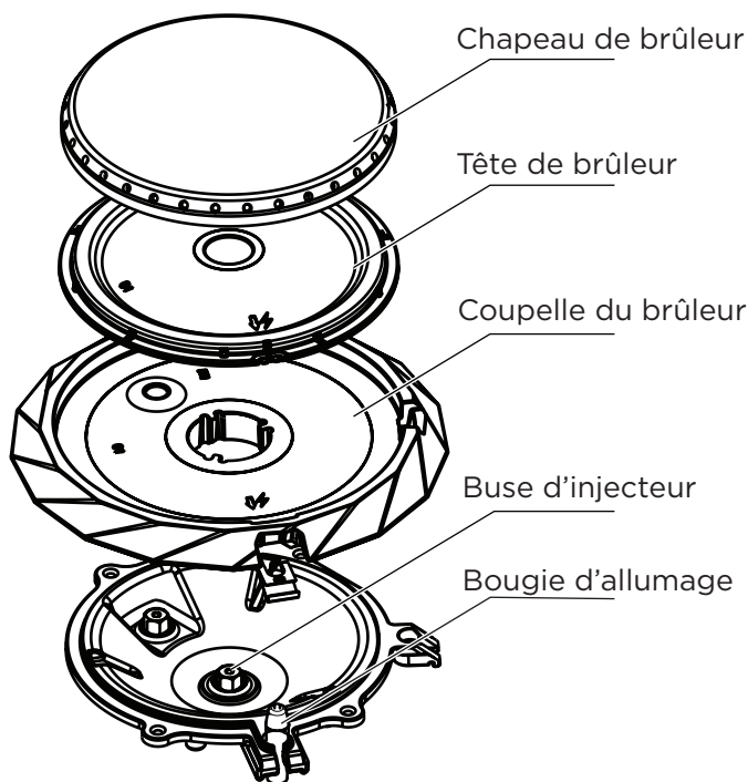
Figure 2: Double brûleur
