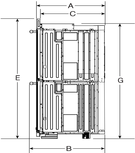
VISTA LATERAL
