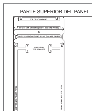
Plantilla de panel de puerta personalizado
