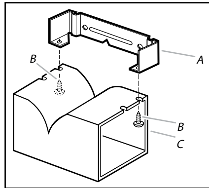
A. Soporte de la cubierta del ducto B. Tornillos de 2,9 x 6,5 mm C. Desviador D. Ducto de escape
