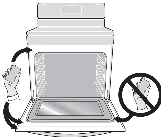
Figure 11: Nettoyer le pourtour du joint de la porte du four
