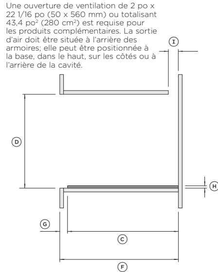
ÉLÉVATION LATÉRALE avec les panneaux avant
