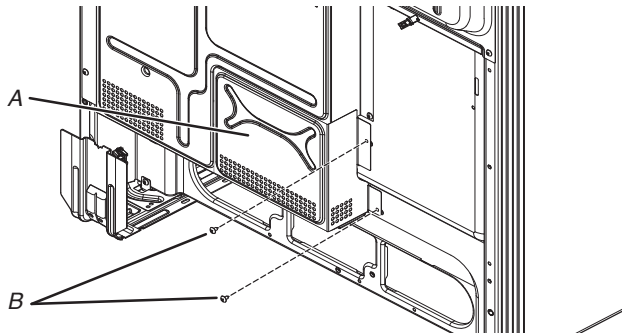
A. Tapa del bloque de terminales B. Tornillos (2)
