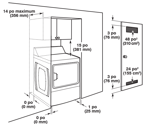
Installation dans une armoire
