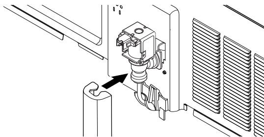
Installation du bouclier de l'électrovanne d'eau
