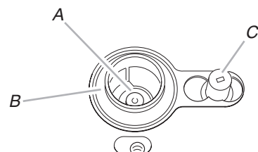
A. Injecteur B. Support d'injecteur C. Électrode d'étincelle
