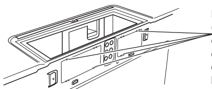
Panneau arrière du four
