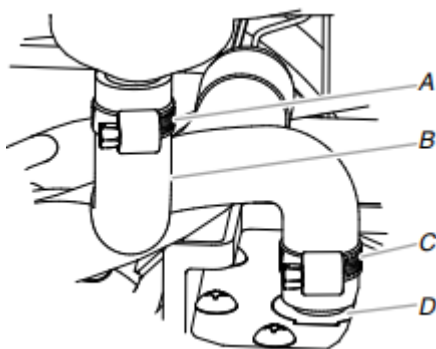
A. Bride de tuyau réglable de 7/8 po B. Tube de vidange (entre le bac à glaçons et la pompe de vidange) C. Bride de tuyau réglable de 7/8 po D. Entrée du réservoir de la pompe de vidange
