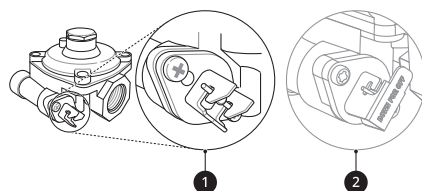
① Posición abierta de la palanca
