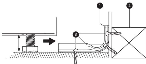
① Soporte antivuelco
