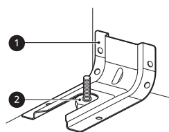
① Soporte antivuelco
