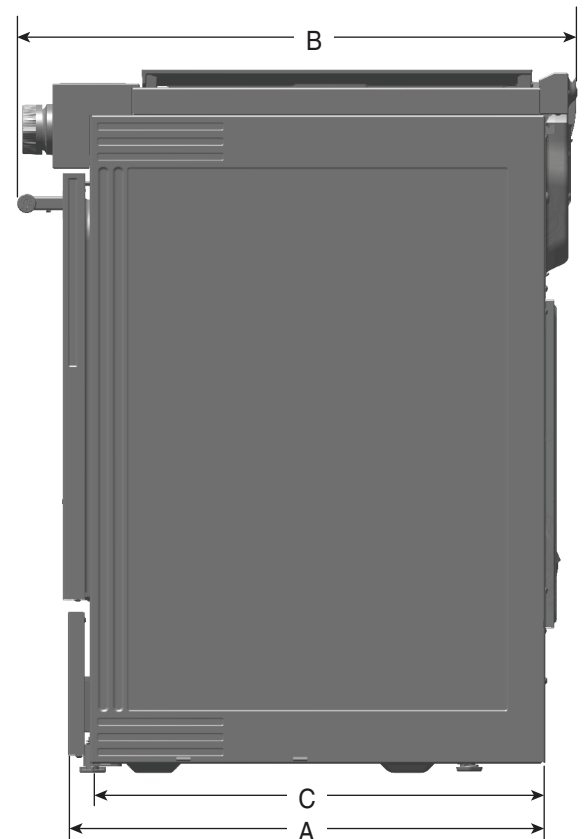
VUE LATÉRALE
