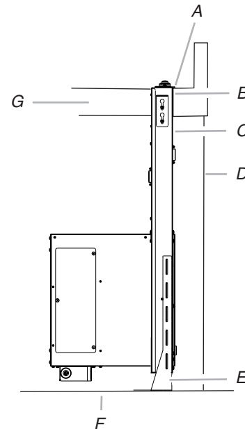
A. Rebord arrière du système d'extraction par le bas
