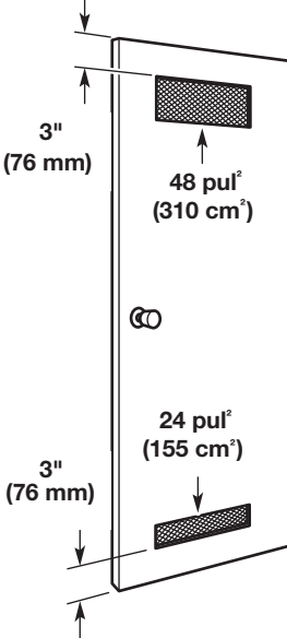
Tamaños mínimos aceptables de los ductos de la puerta del clóset
