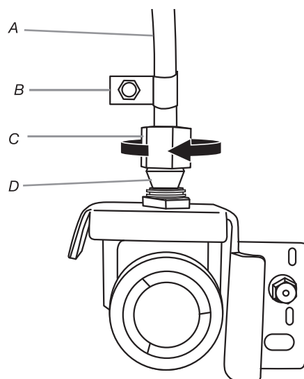
A. Tuyau en cuivre ou en polyéthylène réticulé B. Bride en « P » C. Écrou à compression D. Bague de compression
