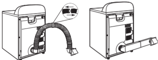
Installation au-dessus de la sècheuse (également offerte avec un coude décalé). L'exemple suivant présente un système d'extraction semi-rigide. Installation en périscope
