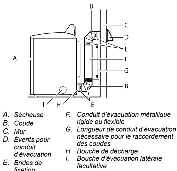
Installation au-dessus de la sécheuse (également offerte avec un coude décalé) Installation en périscope
