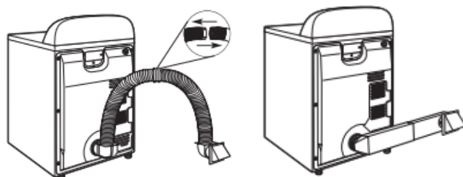
Installation au-dessus de la sécheuse (également offerte avec un coude décalé) Installation en périscope
