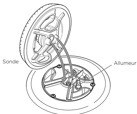
Positionnement correct du diffuseur de flamme - brûleur double
