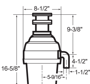
GFB760N
