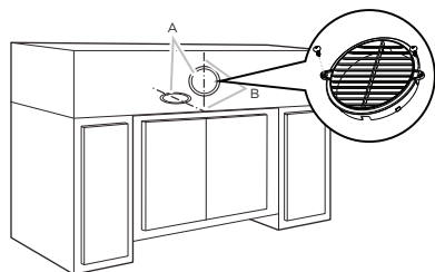
A. Vent cover B. Centerline
