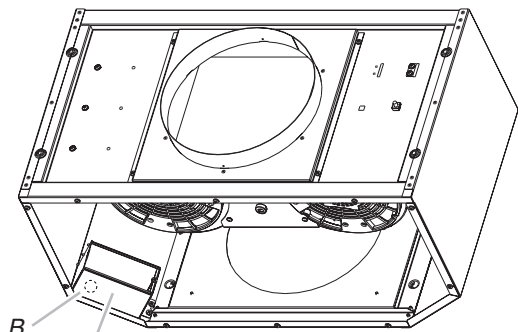
A. Boîtier de connexion électrique B. Opercule arrachable
