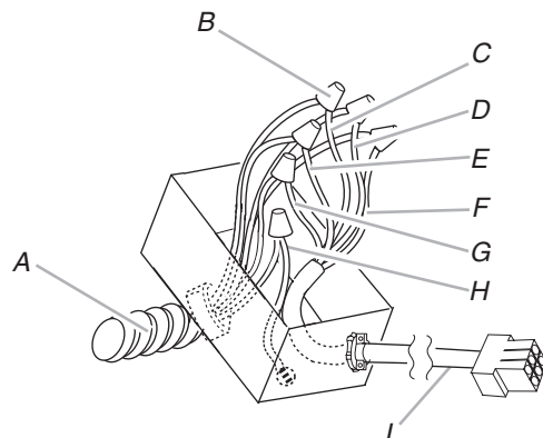
A. Conduit de câblage de 1/2" (1,3 cm) homologué UL ou CSA B. Connecteurs de fils (homologation UL) C. Conducteurs noirs D. Conducteurs blancs E. Conducteurs rouges
